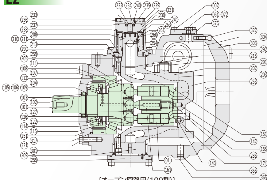
〔オープン回路用(100型)〕 for Open circuit
