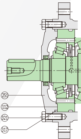
LX-500の場合 in case of LX-500
