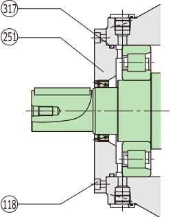
LXV500の場合 in case of LXV500
