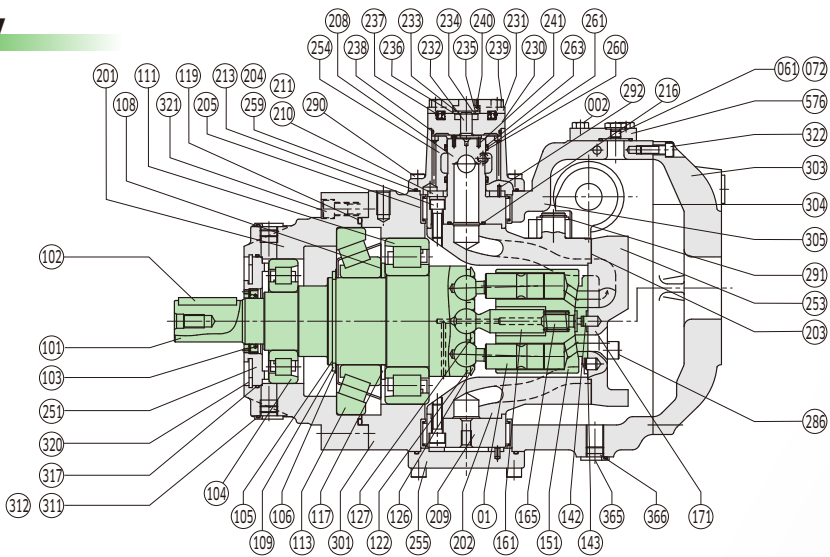
〔オープン回路用(100型)〕 for open circuit
