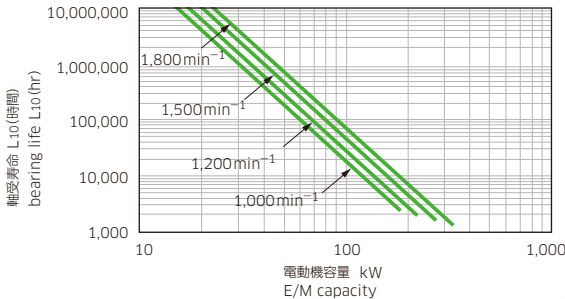
◆軸受寿命 Bearing life
