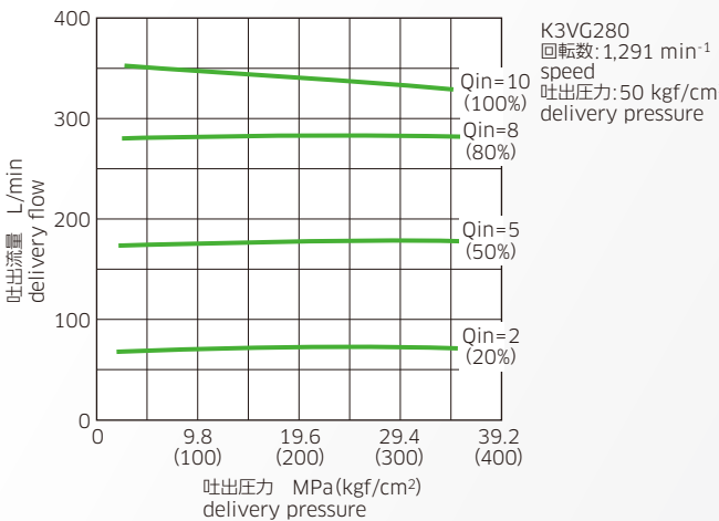
◆圧力-流量特性 Pressure-flow characteristics
