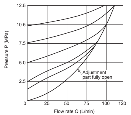
●RD 10 8 /100
